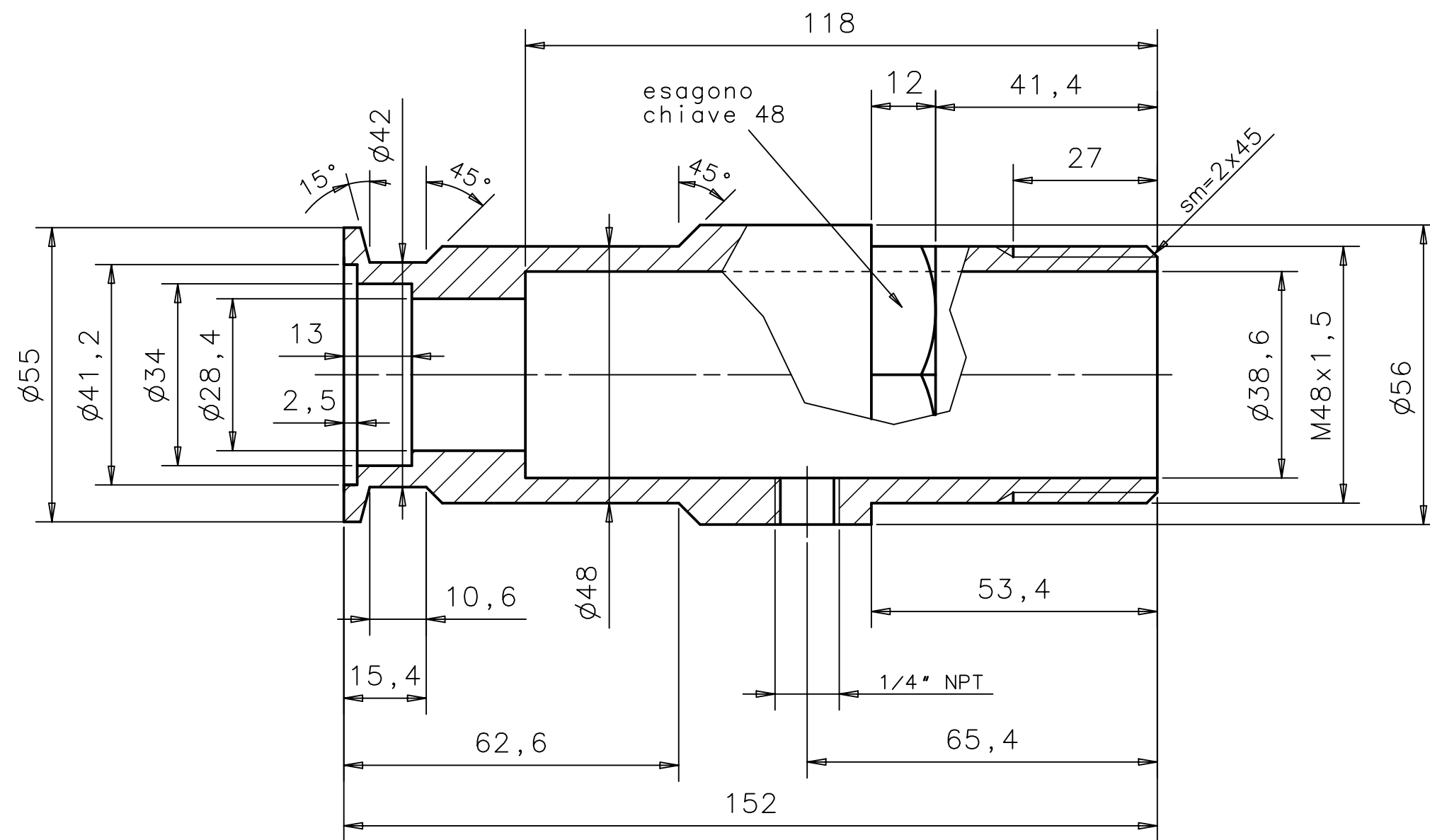
Sez. A-A
