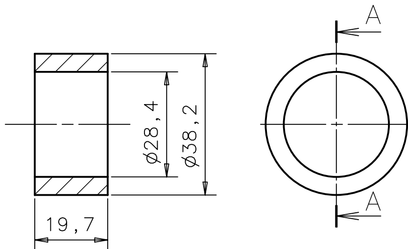
Sez. A-A
