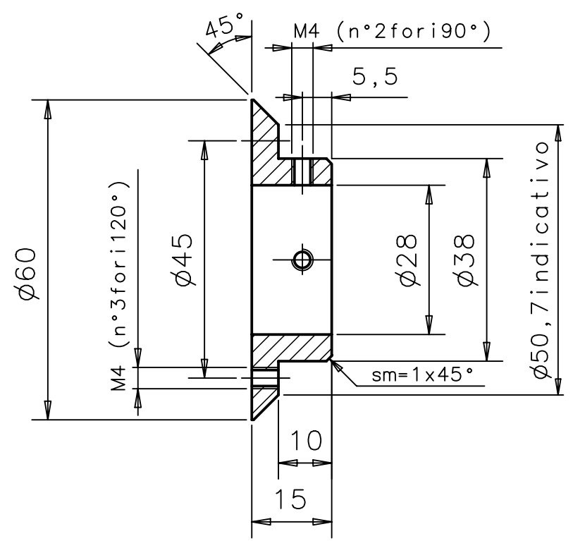
Sez. A-A
