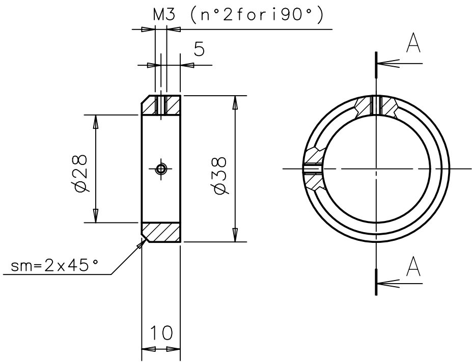
Sez. A-A
