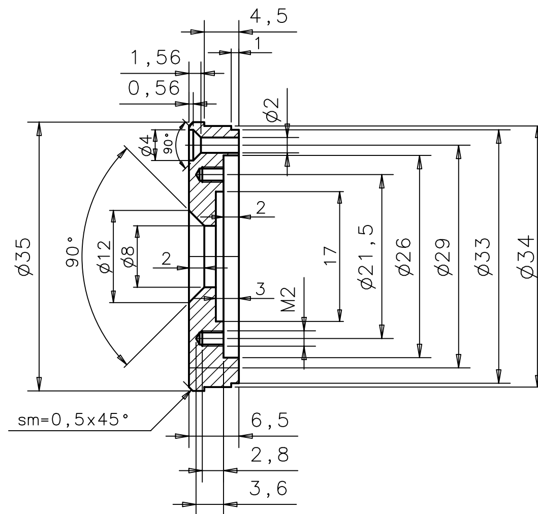
Sez. A-A
