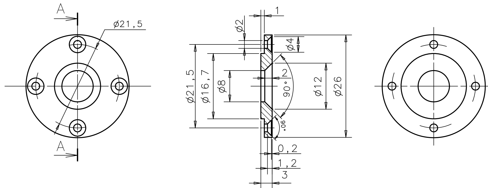
Sez. A-A
