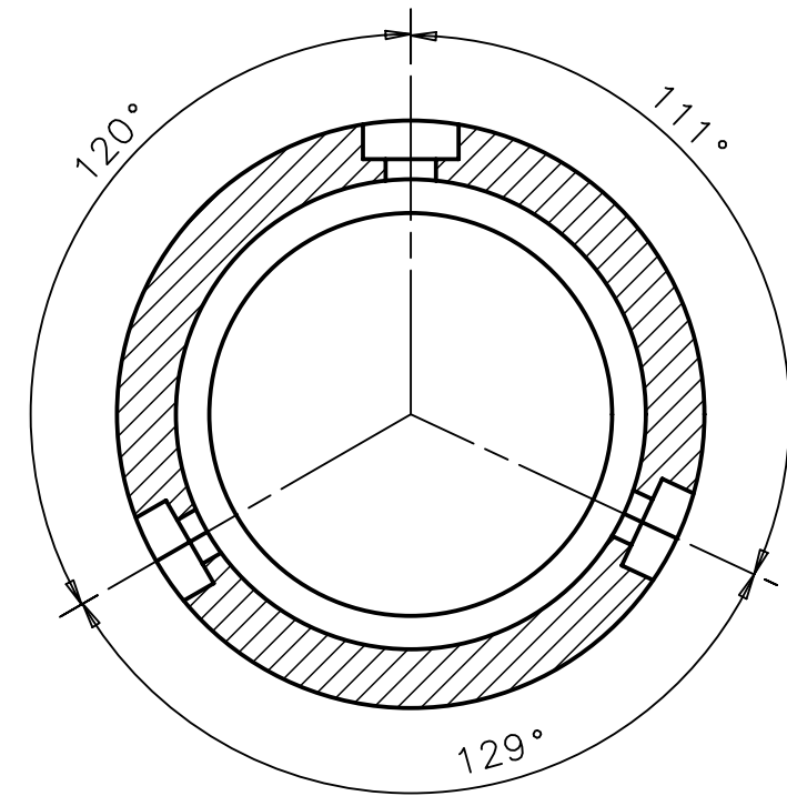
Sez. A-A
