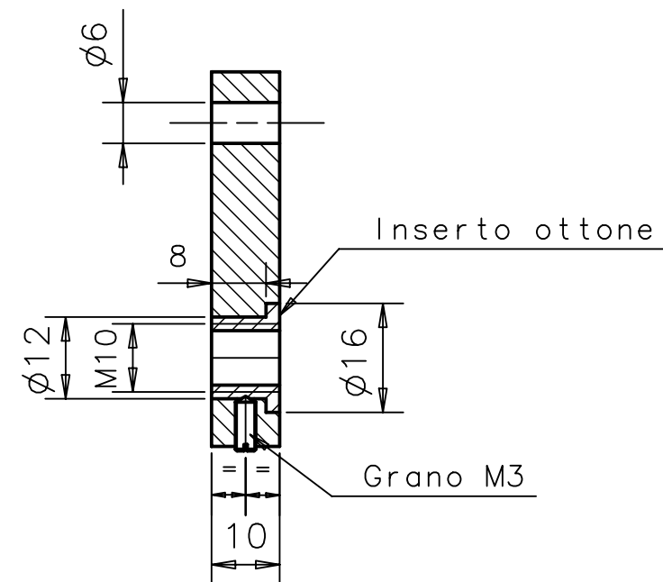
Sez. A-A
