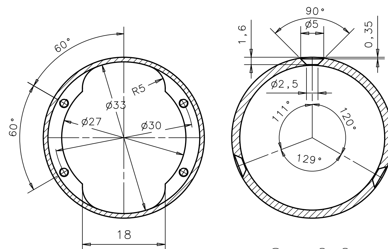
Sez. C-C
