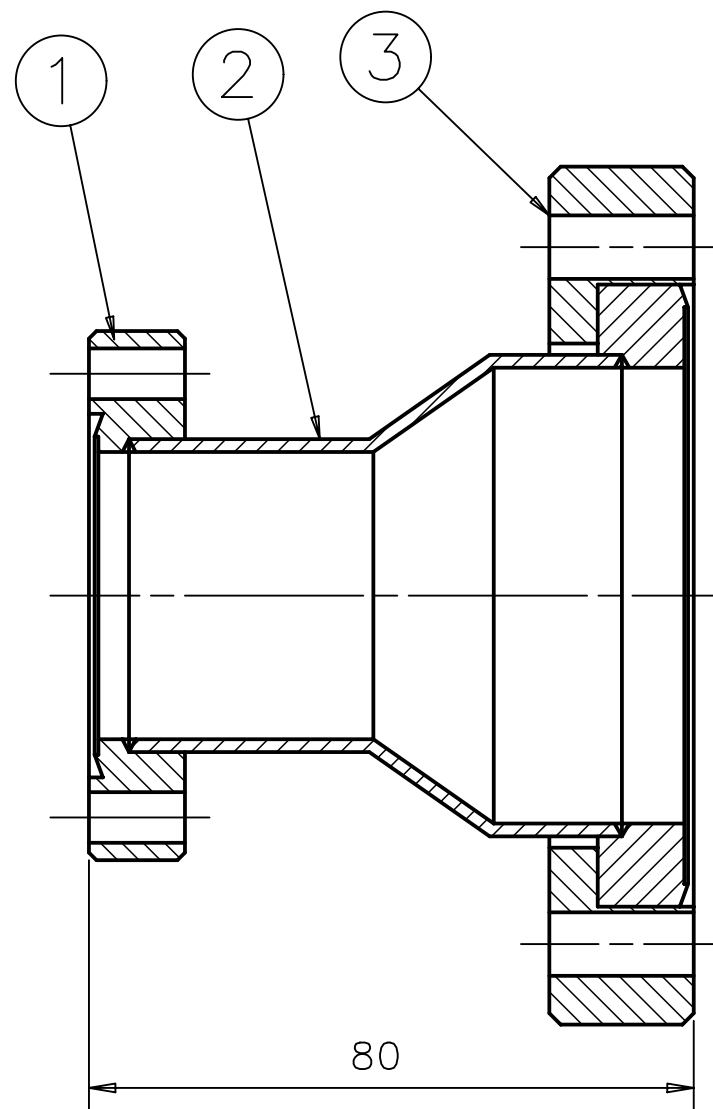
Sez. A-A
