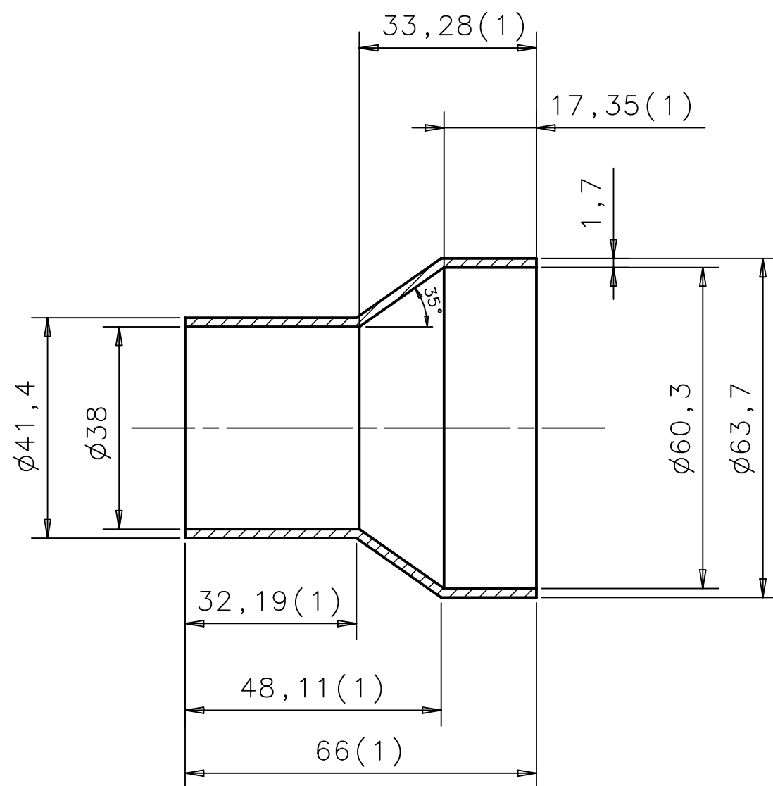
Sez. A-A
